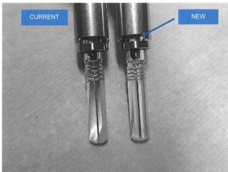
図1 現行品(P/N237306)と新しくラベルが付けられた陰極
